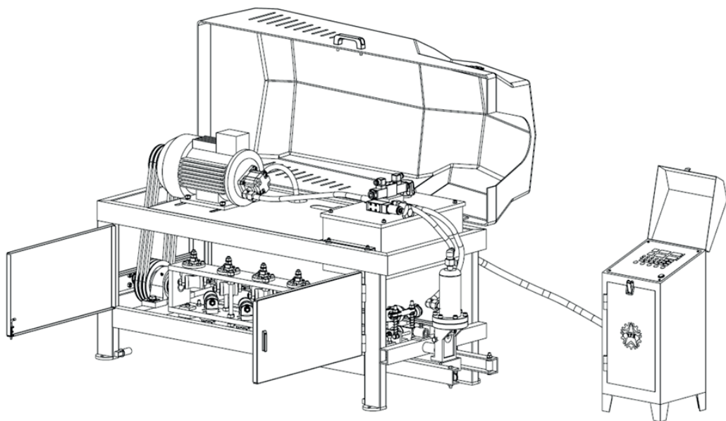
Рис. 1. Схема устройства правильно-отрезного станка VPK ПРО-14К: 1 – рама станка, 2 – электродвигатель, 3 – масляный насос, 4 – масляный бак, 5 – пульт управления, 6 – гидропривод ножа, 7 – подвижная каретка, 8 – узел счетчика длины, 9 – правильная рама.
