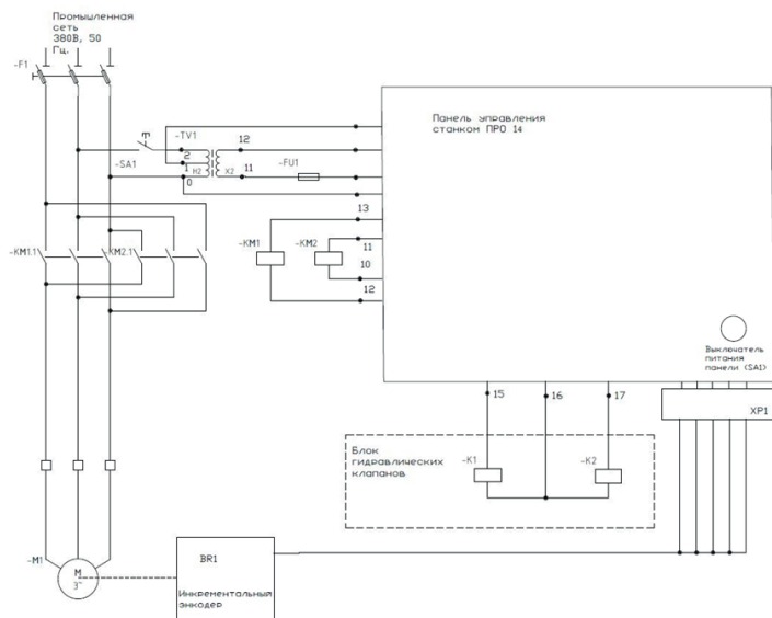
Рис. 4. Принципиальная электрическая схема станка VPK ПРО-14К.
