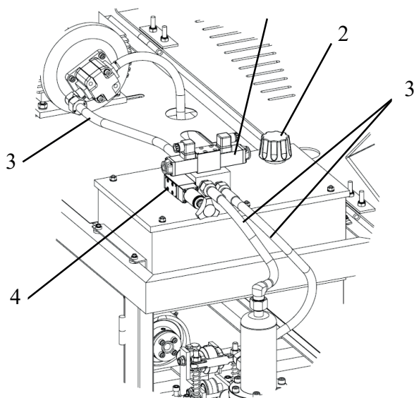
Рис. 3. Гидросистема: 1 – электромагнитный клапан, 2 – заливная горловина, 3 – рукава высокого давления, 4 – гидравлический предохранительный клапан.
